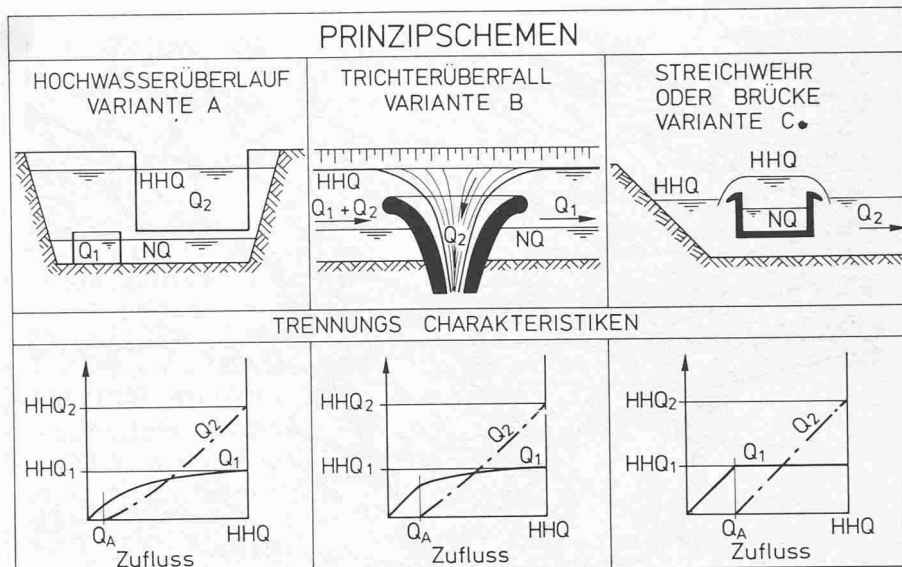
Bild 3. Prinzipischemen für drei mögliche Varianten von Verzweigungsbauwerken und deren Abflusscharakteristiken für Q_1 und Q_2
