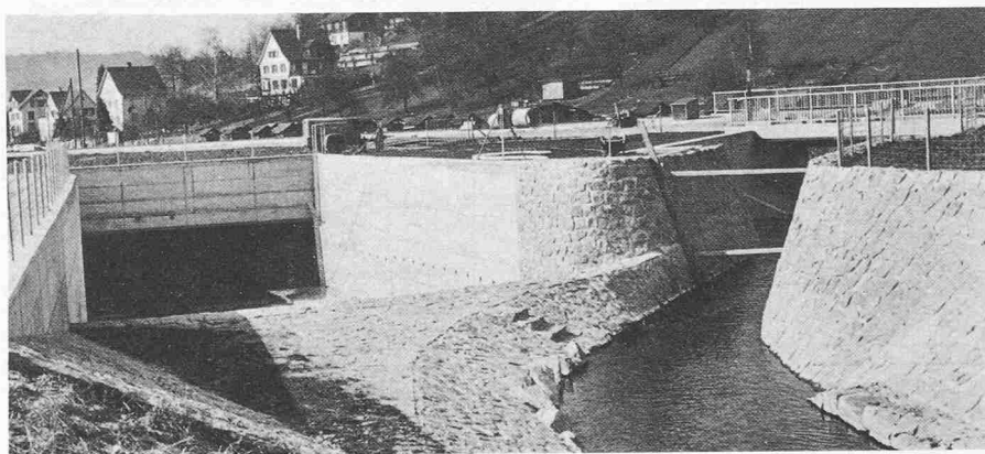
Bild 4. Verzweigungsbauwerk der Eulach bei Hegi. Der breite Hochwasserüberlauf (links) entlastet die Hochwasserspitze über ein Tosbecken in den überdeckten Umleitstollen mit Freispiegelabfluss. Nach dem Wassersprung im Tosbecken stellt sich im Stollen ein strömender Abflusszustand ein. Rechts ist die Überleitung in den alten Eulachlauf sichtbar. Die auf Winkeleisen geschraubte Tauchwand zur Abweisung von Gschwemmsel sowie zur Reduktion der Wassermenge im alten Lauf ( Q_1 ) ist noch nicht montiert
