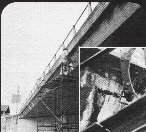
Risse in Betonbauwerken Abdichtung mit Renesco- Flexin-Injektionen
