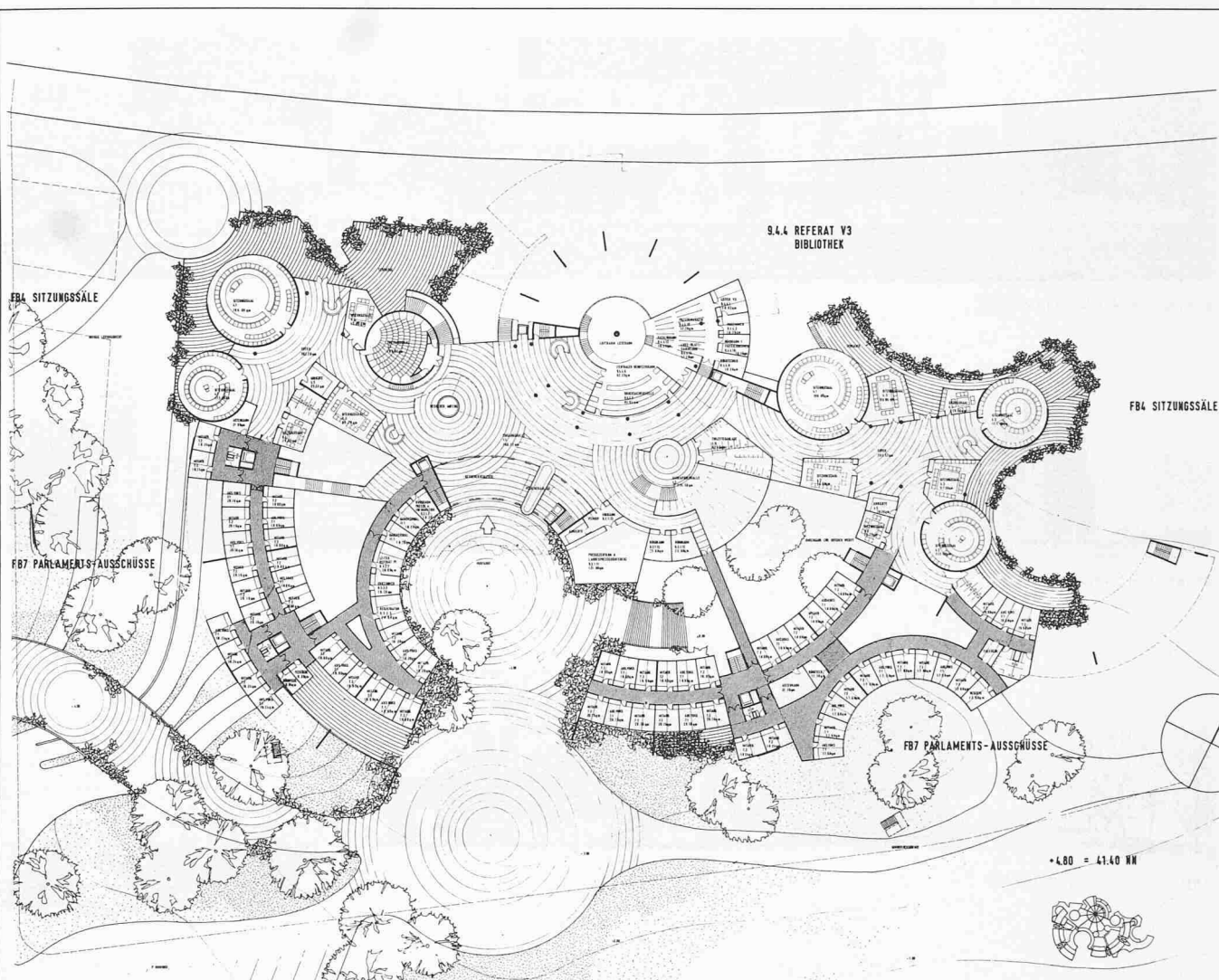
Grundriss 1. Obergeschoss 1:1100
