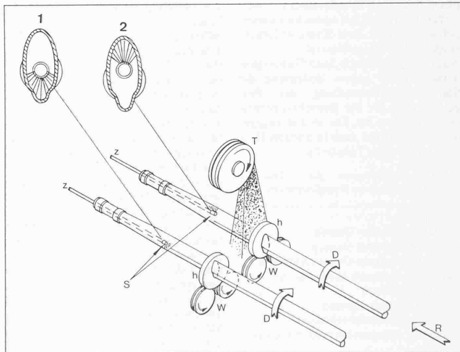
Bild 16. Arbeitsprinzip der Wheelabrator-Anlage zum Peenen der Helikopter-Propeller in den Werken der Boeing Comp., Vertol Division, mit Schleuderrad zur Behandlung der Aussenfläche, während die Wurzelenden mit Druckluft-Strahldüsen gepeent werden. W: Auflagerollen der vier Walzen zur Aufnahme von zwei nebeneinanderliegenden Propellerblättern; D: Drehrichtung der Propellerblätter auf dem Werkstückwagen; R: Vorschubrichtung des Werkstückwagens mit den darauf liegenden Propellerblättern; S: nach dem Druckluftsystem arbeitende Strahldüsen für das Peenen der Innenseite der Wurzelenden.
