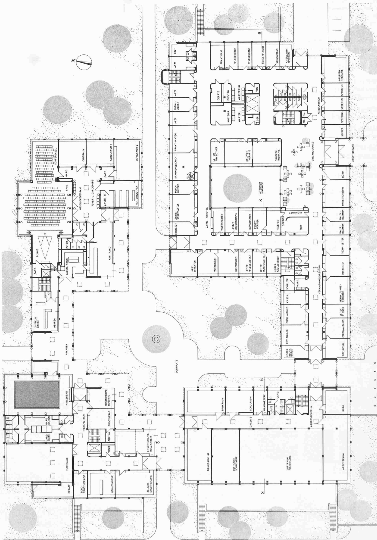
Zentrum Erdgeschoss 1:500
