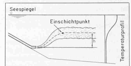
Bild 6. Einleitung von gereinigtem Abwasser in einen See während der Sommerstagnationsperiode. Infolge der Einmischung von Seewasser kann der Abwasserstrahl seinen Auftrieb verlieren und sich ein-schichten , ohne an die Seeoberfläche aufzusteigen
