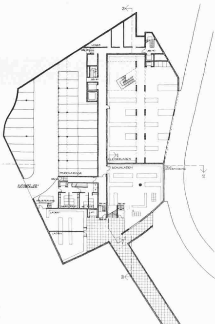
Grundriss 1. Untergeschoss 1:1000
