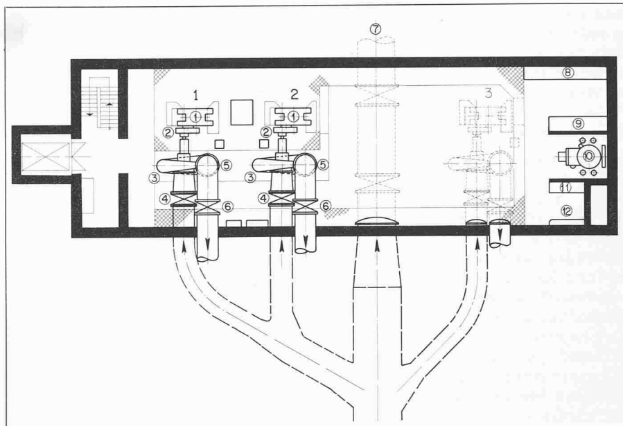
Bild 9. Grundriss Zubringerpumpengeschoss
