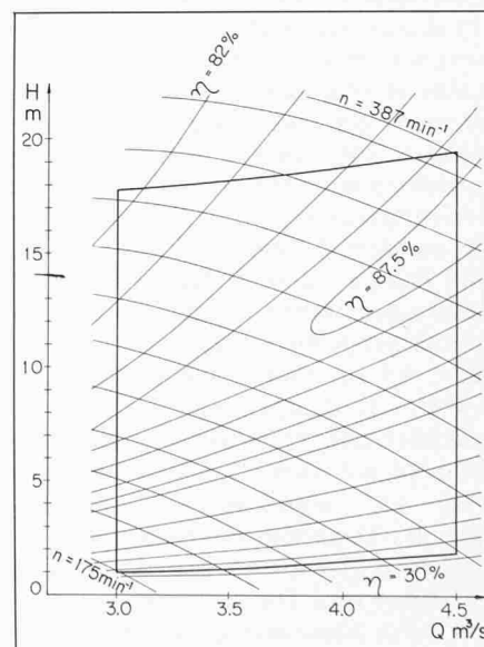
Bild 10. Charakteristiken der Zubringerpumpen
