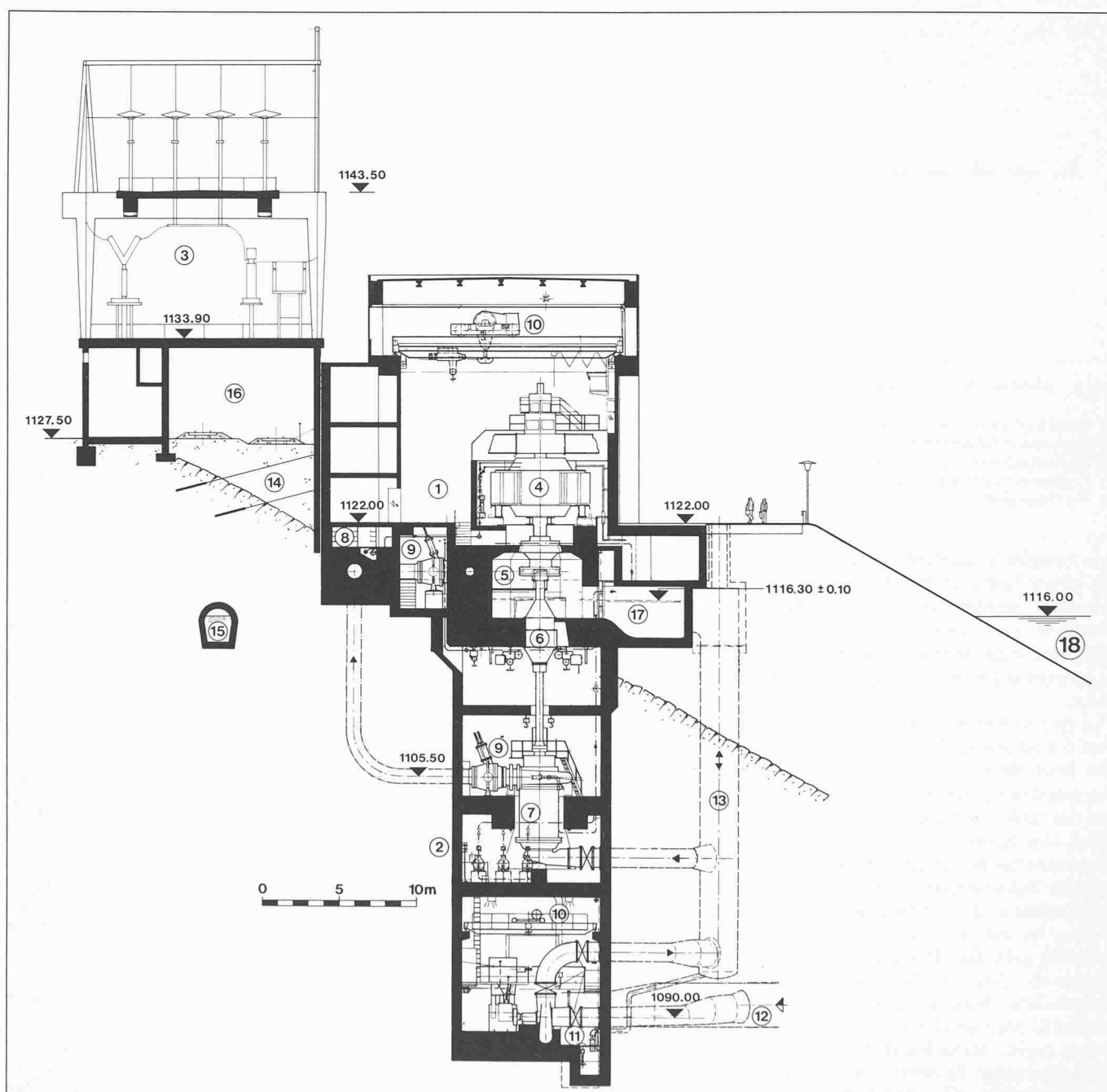
Bild 4. Zentrale Châtelard II. Vertikalschnitt
