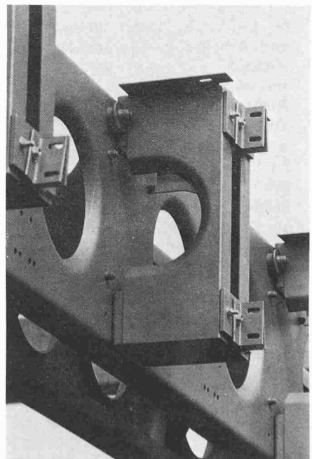
Detail Fassadenkonsole
