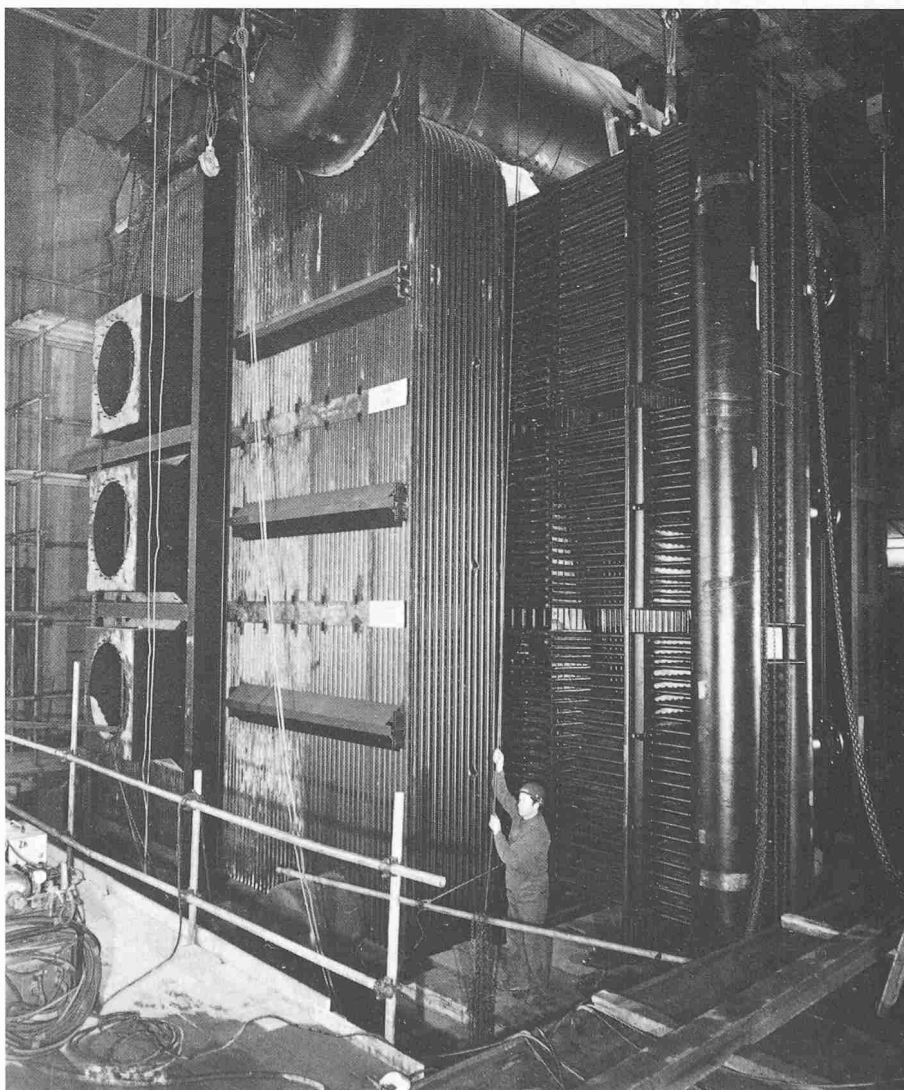
Bild 16. Sulzer-2 Trommel-Strahlungskessel, Frontansicht mit Brennergehäusen und Überhitzer vor Einbau
