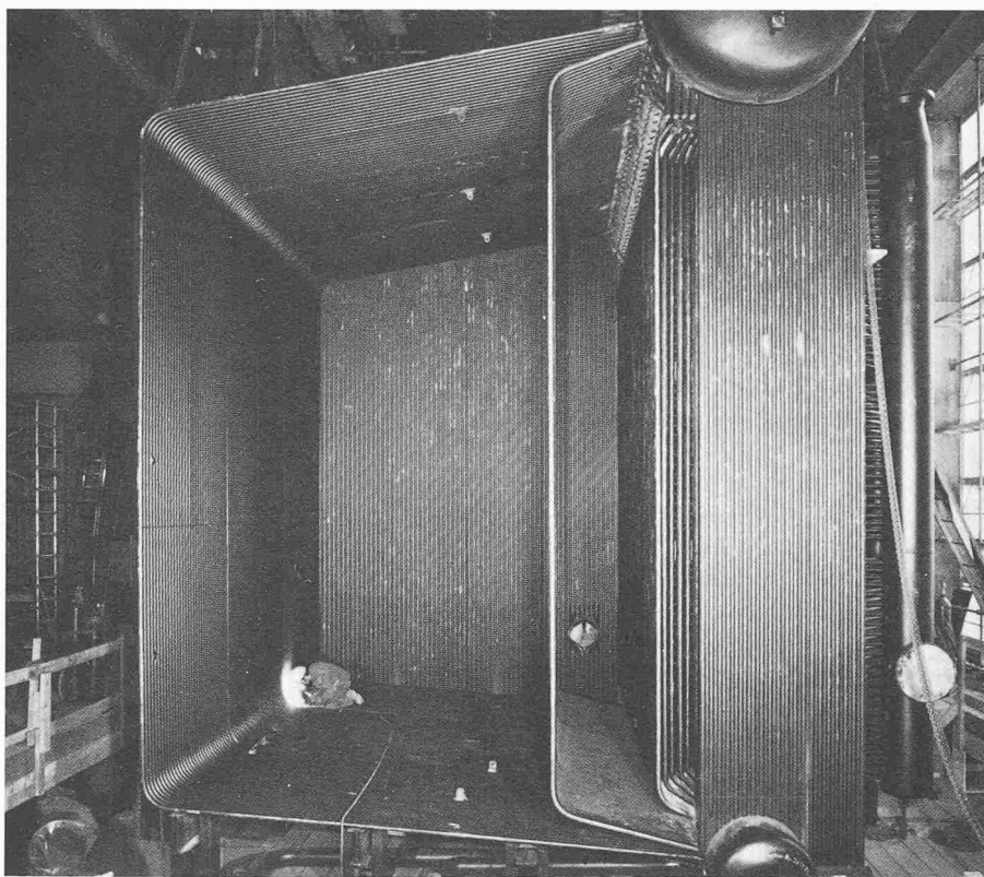
Bild 15. Sulzer-2 Trommel-Strahlungskessel, Typ ZL, Leistung 100 t/h, Druck 25 bar, Temperatur 245 °C. Blick in Brennkammer und Leerzug, Frontwand noch nicht montiert
