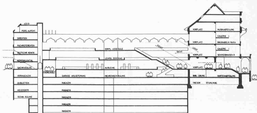
Schnitte 1:850
