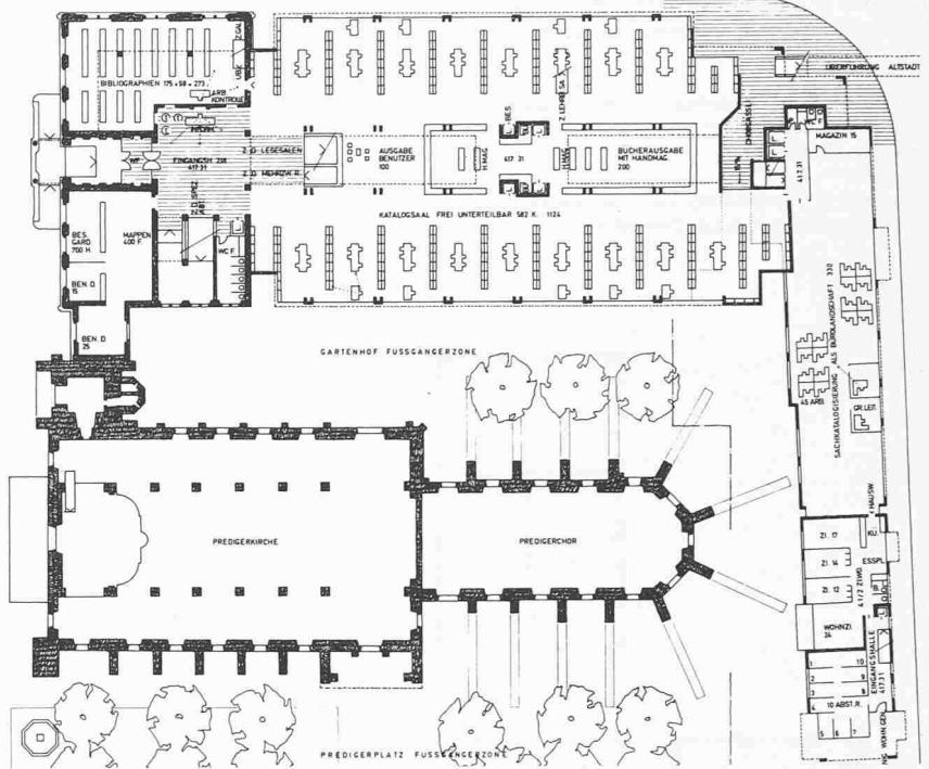
Geschossebene Seilergraben 1:850
