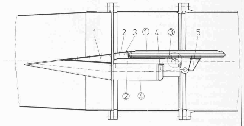
Bild 3. Schwenklappe. 1 Drehteller, 2 Querträger, 3 Abstützung, 4 Servomotor, 1 + 5 Strömungskörper
