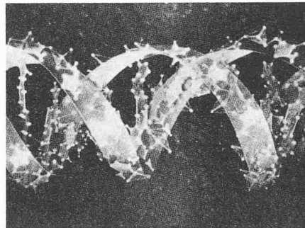
Bild 5. Molekülketten[23]
