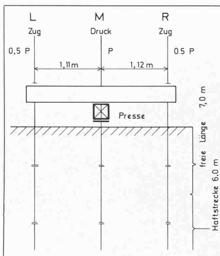
Bild 5. Versuchsanordnung. 1. Versuch
