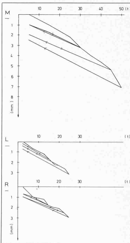
Bild 6. Last-Setzungsdiagramm. 1. Versuch
