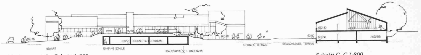
Nordwestansicht, Schnitt 1:800
