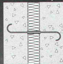
Zuganker
