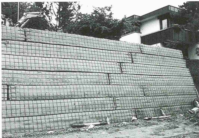
Geogreen-Stützmauersystem
