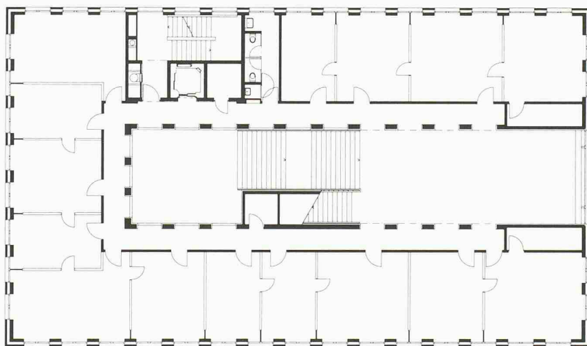
1. Obergeschoss
