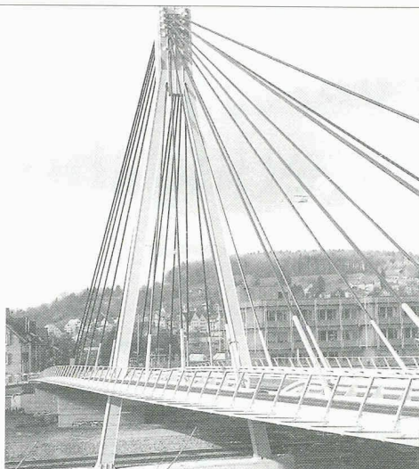
Projekt: Storchbrücke Winterthur Ingenieure: Höltschli + Schürter, Oberflikon
