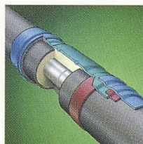
Nachisolierrsysteme
