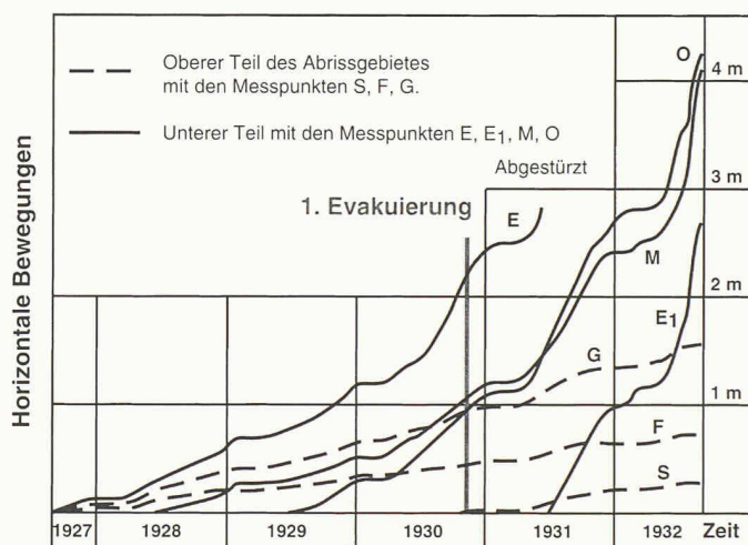
3 Horizontale Bewegungen verschiedener Messpunkte im Abrissgebiet des Kilchenstocks in der Zeitperiode 1927–1932 (nach [1])
