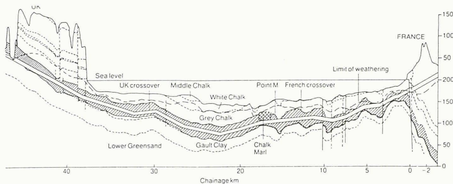
Geologisches Längsprofil des Ärmelkanaltunnels (aus [11])
