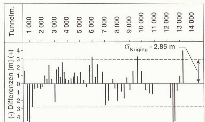
Differenzen tatsächlicher Tiefenlage minus Prognose der Basis der Kreidekalk im französischen Abschnitt des Ärmelkanaltunnels (nach [10])
