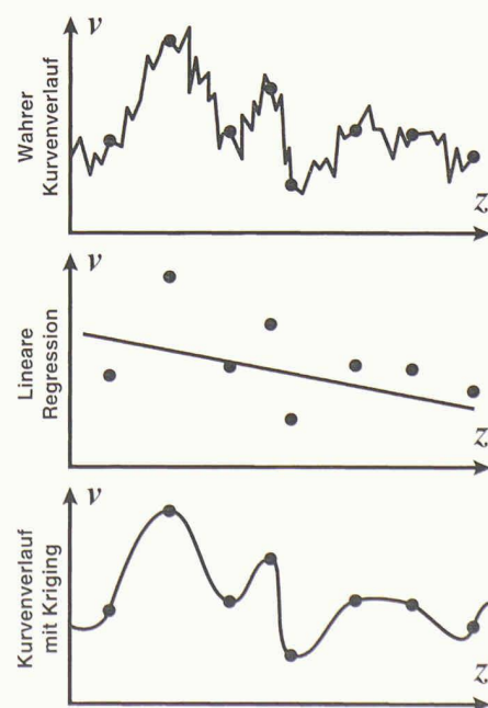
Natürliche eindimensionale geologische Heterogenität mit Stützpunkten (oben), lineare Interpolation (Mitte) und Schätzung mittels Kriging (unten)
