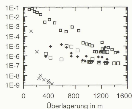
Korrelationsdiagramme der Gebirgsüberlagerung mit den Transmissivitäten 100 m langer Tunnelabschnitte im zentralen Aaregranit (links) und dem südlichen Altkristallin des Gotthard-«Massivs» (rechts). Die verschiedenen Symbole kennzeichnen unterschiedliche Tunnel
