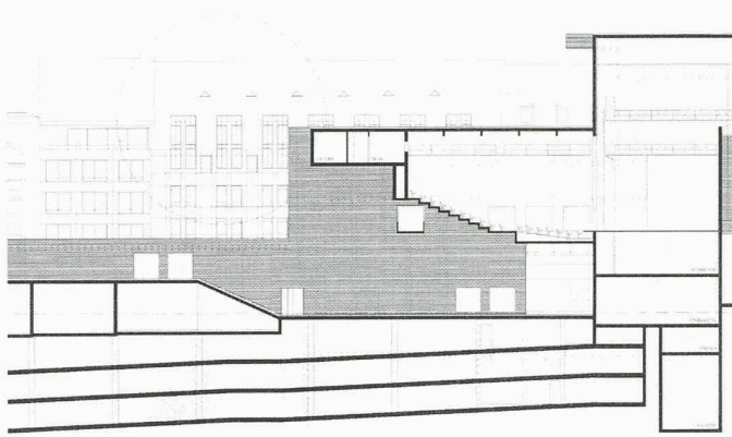
Projekt von Jakob Steib. Längsschnitt durch das Theatergebäude. Blick Richtung Westen
