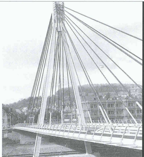
Projekt: Störchenbrücke Winterthur Ingenieure: Höltschi + Schürter, Oerlikon
