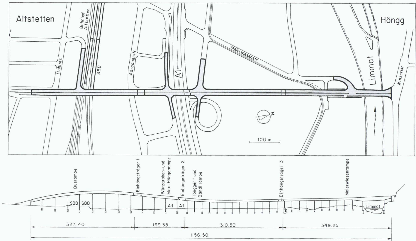
Europabrücke – Situation und Längsschnitt (überhöht)
