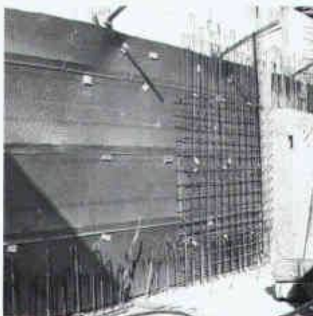
Filter- und Sickerschicht, keine Baugrubenverfüllung!
