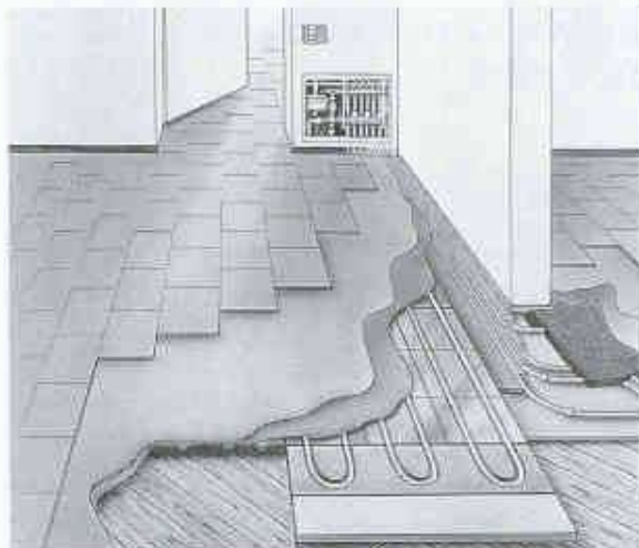
Stramax-Fussbodenheizung von Gebrüder Tobler AG
