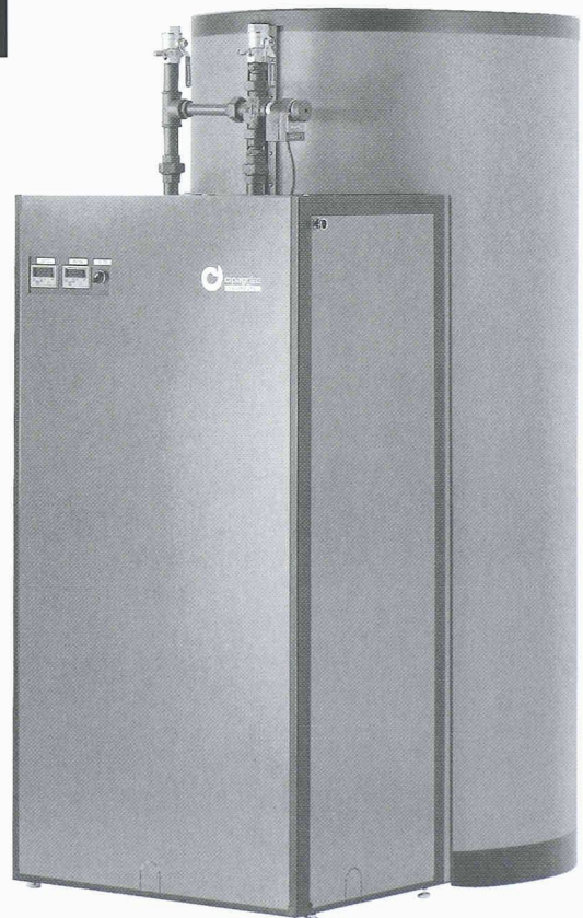
"Kluge", anschlussfertige Warmwasser- produktions-Einheit Cipag-variobloc (15 Modelle von 400 bis 1000 Liter).
