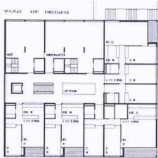
Wohnhaus Erdgeschoss
