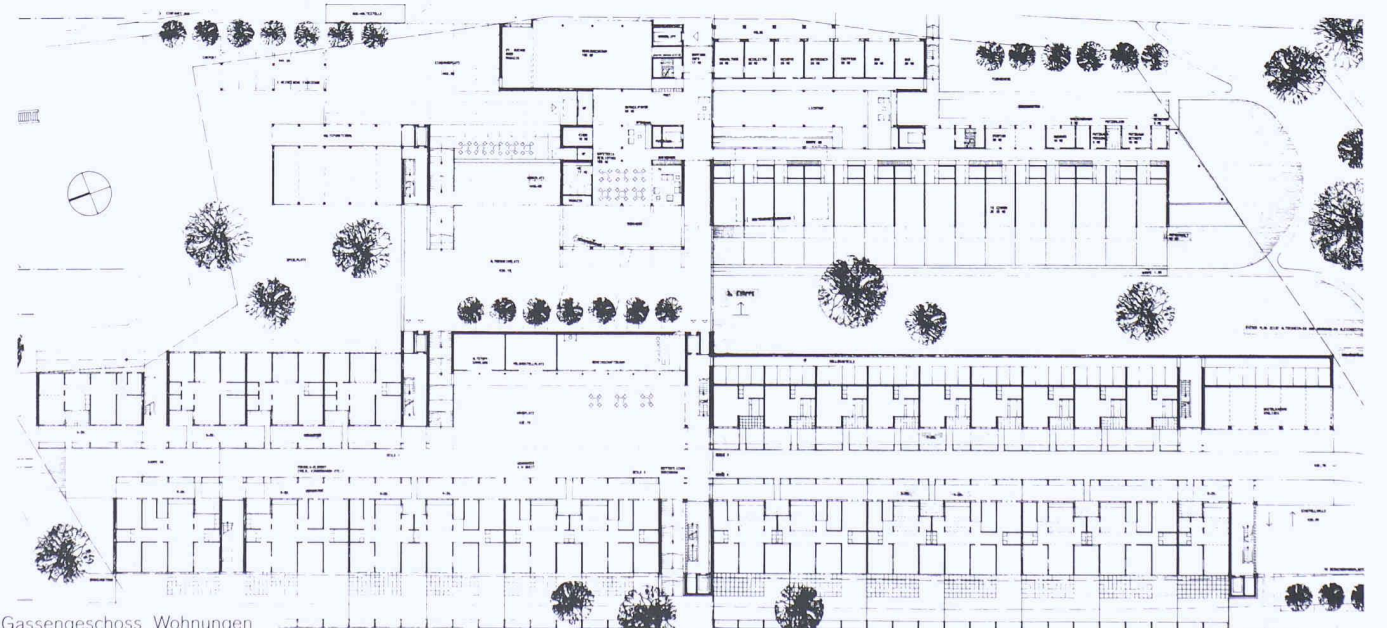
Gassengeschoss Wohnungen
