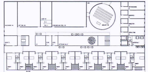
3. Obergeschoss
