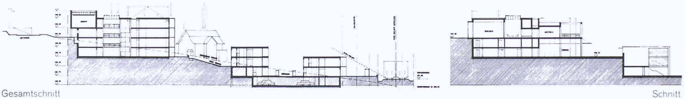
Gesamtschnitt
