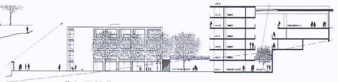
Schnitt Halle
