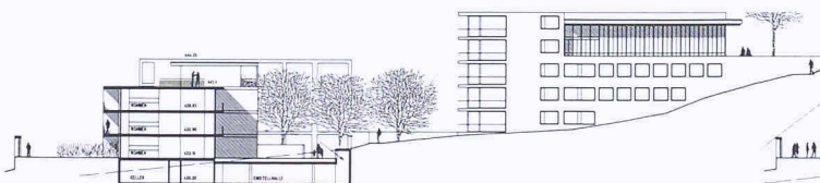
Schnitt Wohnzeile
