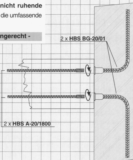
Grundriss-Detail
