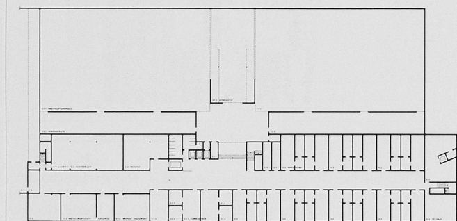
Untergeschoss
