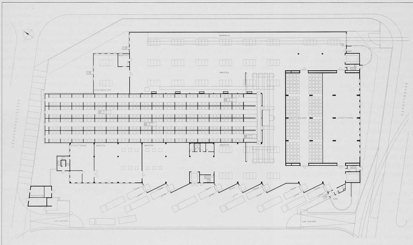
Bild 3. Grundriss Erdgeschoss
