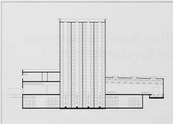
Bild 4. Schnitt durch das Hochregallager
