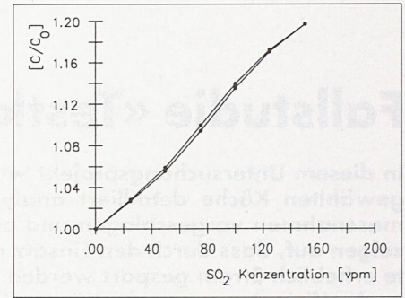
Bild 10. Elektrische Adsorptionsisotherme (SO 2 in trockenem Stickstoff) eines beschichteten Interdigitalkondensators (Heteropolysiloxanschicht)
