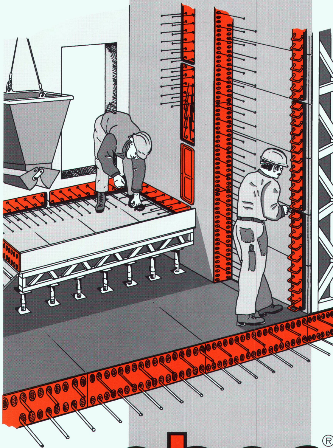
Armierungs- anschlüsse
