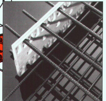
Abschalung
