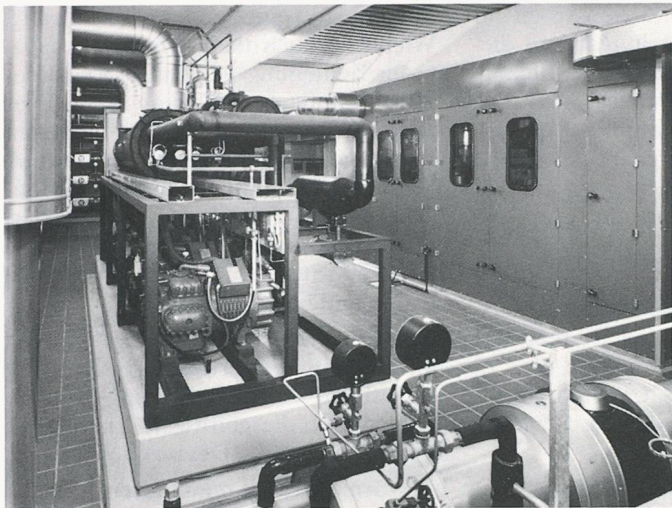
Bild 3. Gas- und Elektrowärmepumpe Wärmезentrale Brugg AG, Zeughaus: links Elektro-Wärmepumpe, rechts geschlossenes Schalldämmgehäuse der Gasmotor-Wärmepumpe (Foto: H. Studer, Postfach 47, 3000 Bern 11)
