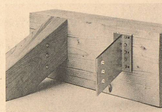
BMF-Balkenträger Alu
