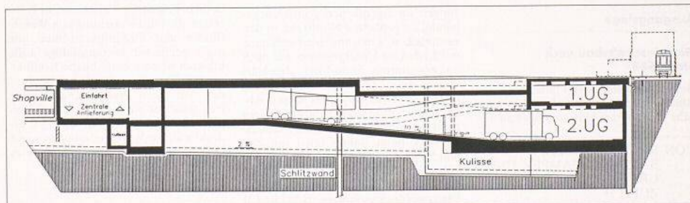
Bild 2. Längsschnitt mit Rampen ins 1. und 2. Untergeschoss
