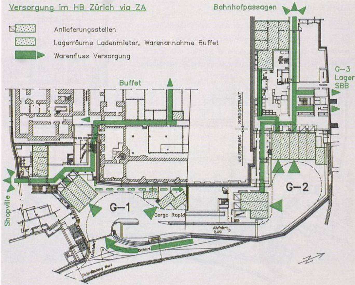
Bild 4. Versorgungsflüsse: Die Warenflüsse zu den Läden im S-Bahnhof, für die Buffetbetriebe und für das Shop-Ville beginnen in der zentralen Anlieferung
