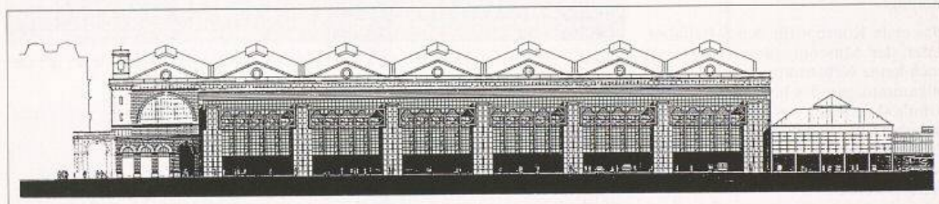
Bild 6. Nordfassade (Seite Landesmuseum) des neuen Nordtrakts mit Türmen und zwischenliegenden Trägern
