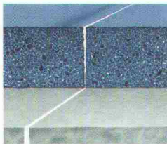
Forschungen der Universität von Nottingham haben bewiesen, dass z.B. Reflektionsrisse durch die Bewehrung mit Tensar AR1 vollständig verhindert werden können.
