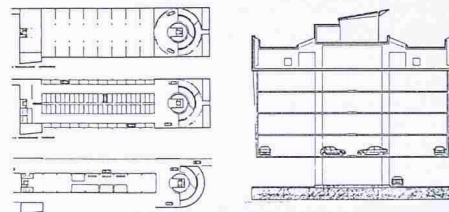
Parkhaus von Christian Coppey
