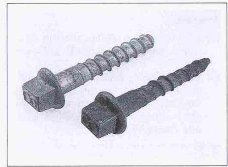
Bild 1. Erhebliche Querschnittsverminderung einer Eisenbahn-Schwellenschraube durch Korrosion
