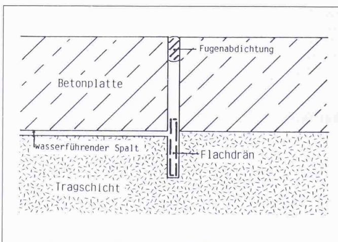
Bild 2. Entwässerung einer Betonfahrbahnplatte durch nachträglichen Einbau von geotextilen Flachdräns. Schnitt durch den Entwässerungsschlitz mit Flachdrän (Wilmers)
