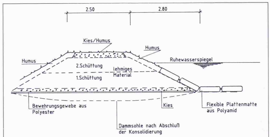
Bild 3. Aussendamm für ein Absetzbecken und Befestigung der Beckensohle mit Plattenmatten aus mit Pumpbeton verfüllter Gewebeschalung (Mohr)
