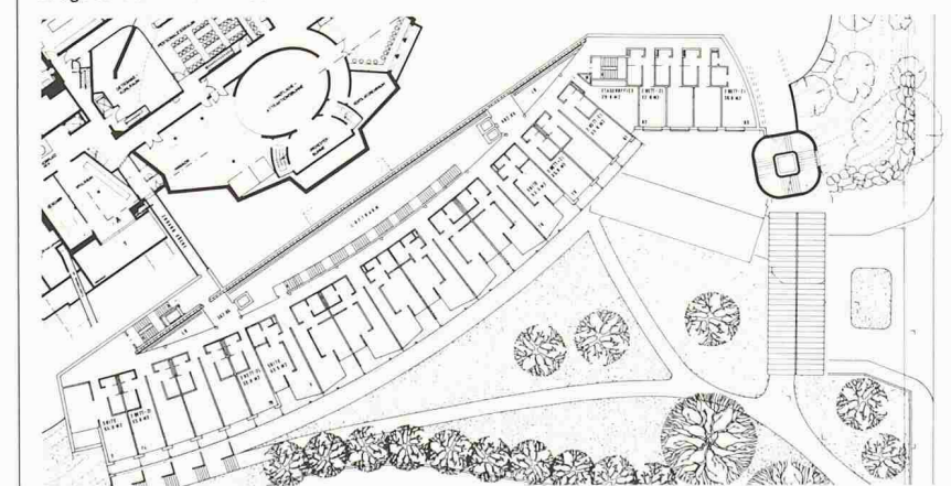
4. Obergeschoss
