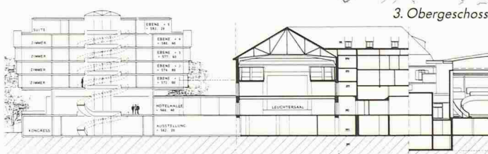
Schnitt
