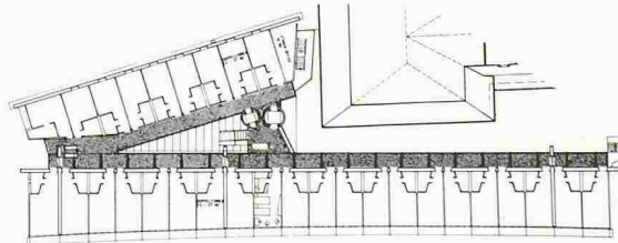
4. Obergeschoss
