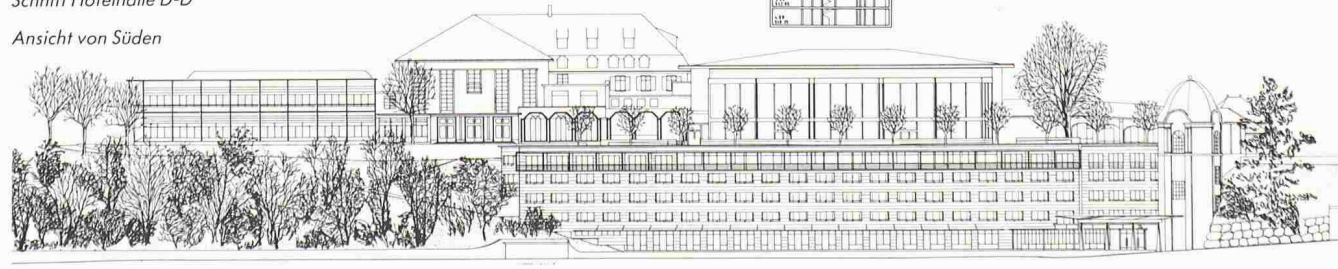
Schnitt Hotelhalle D-D
