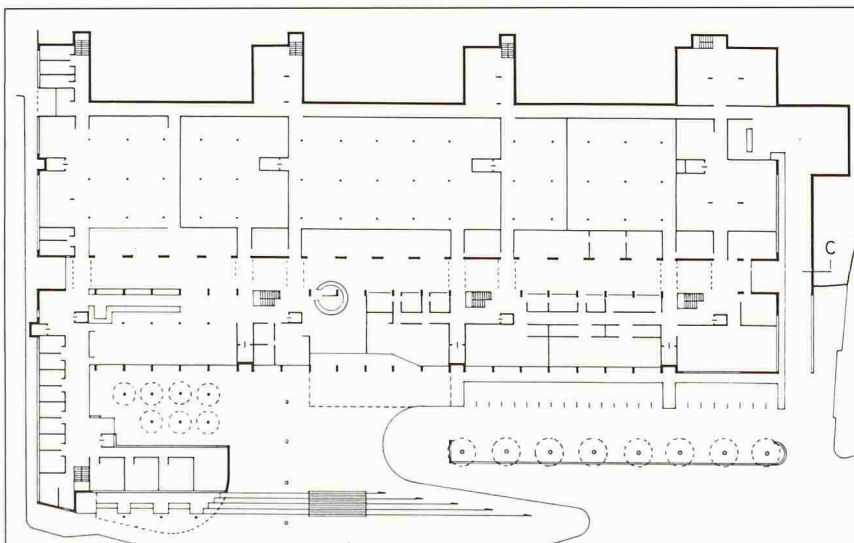
Niveau d'entrée 1:650
