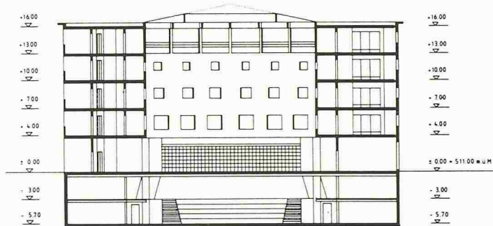
Schnitt B-B
