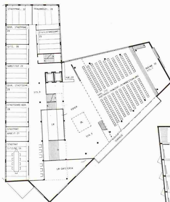
1. Obergeschoss
