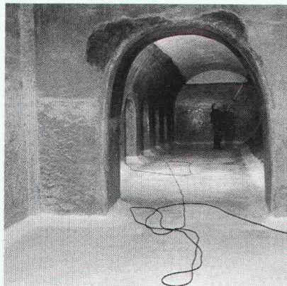
Wasserreservoir Murtenerwald: Kombination von verschiedenen Sanierungs-Methoden: Injektionen gegen eindringendes Wasser und zur Verfestigung des Gewölbes, Auskleidung durch starre Abdichtung.
