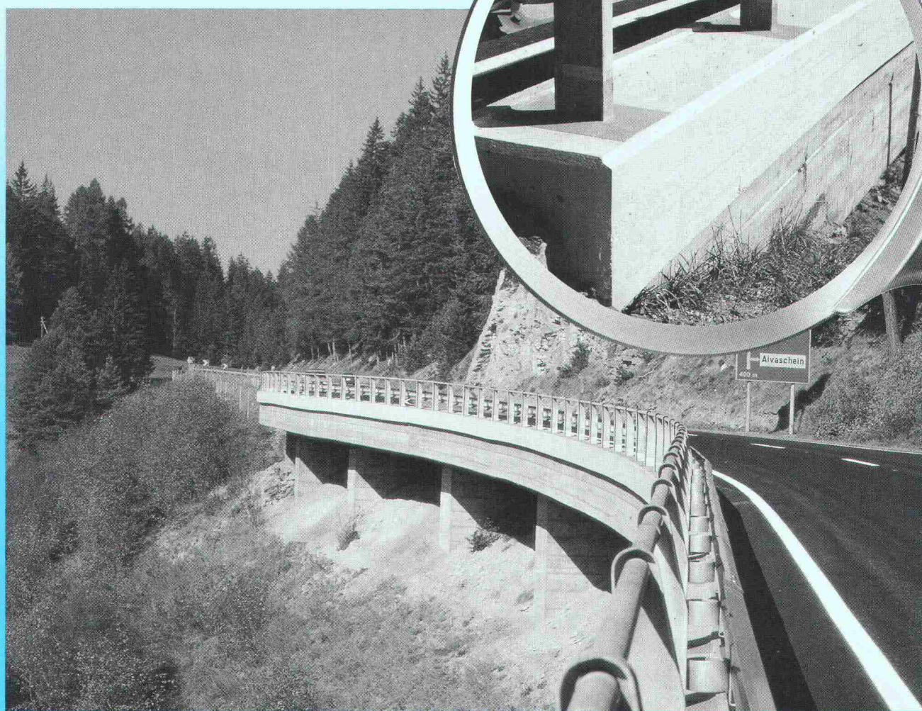
Lehnen-Viadukt, Tiefencastel
