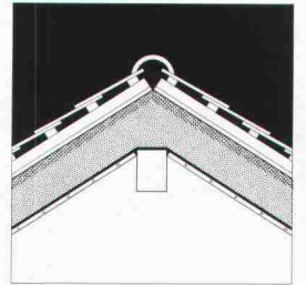
STARTEX in Dachschrägen oder Dachboden
