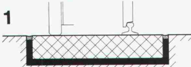
Fahrbahnisolierung
